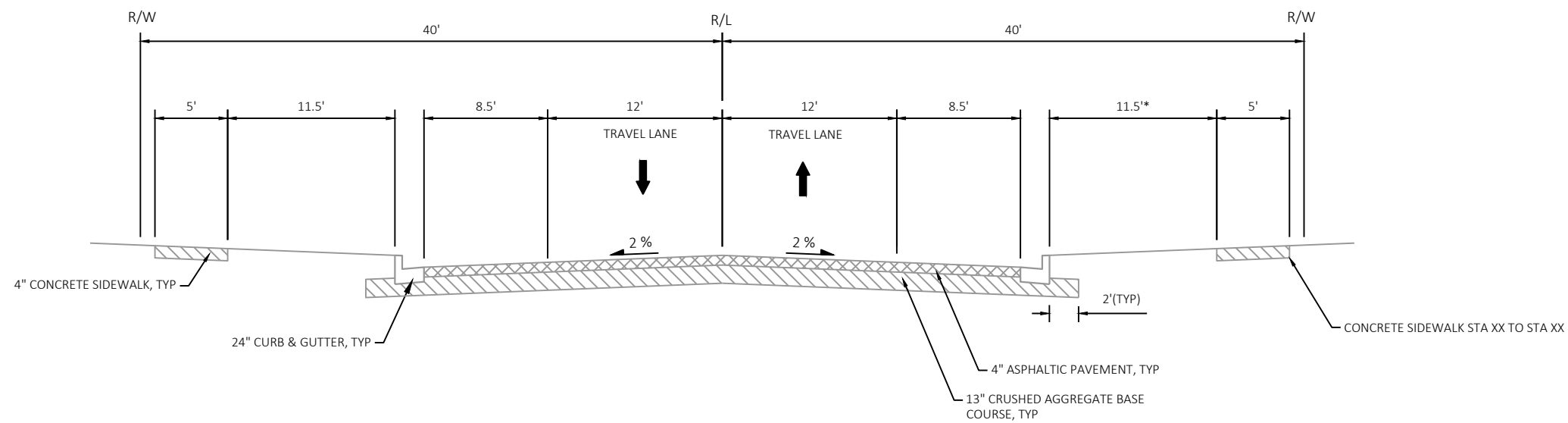
EXISTING TYPICAL SECTION - LIBAL ST STA XX TO STA XX
